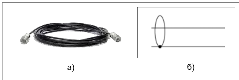
Рис. 12 – Сигнальный кабель: а – внешний вид, б – изображение на схемах
