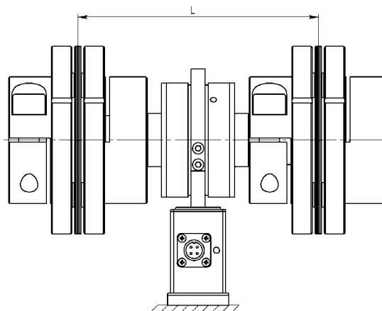
Датчик в сборе с муфтами МВ
