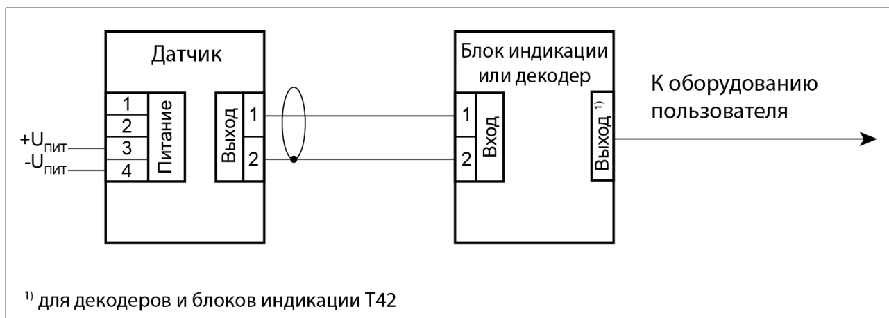
Рис. 13 – Схема подключения датчика М40А к вторичному оборудованию
