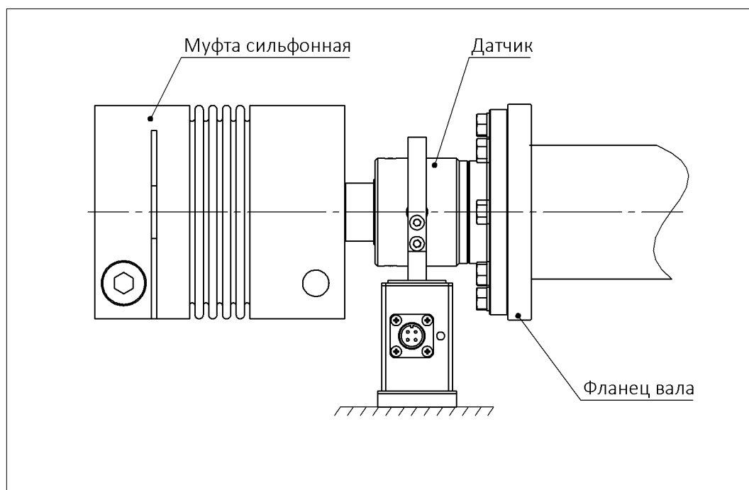
Рис. 8 – Установка датчика М40А с применением сильфонной муфты
