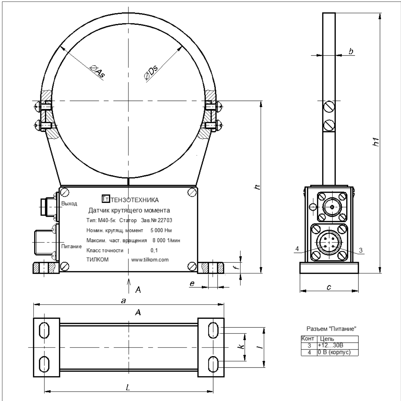
Рис. 7 – Статор М40А-400... М40А-5к. Габаритные и установочные размеры, мм
