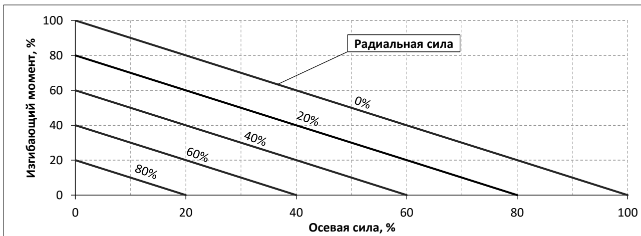
Рис. 4 – Предельно допустимые для датчиков М40А сочетания внешних нагрузок
