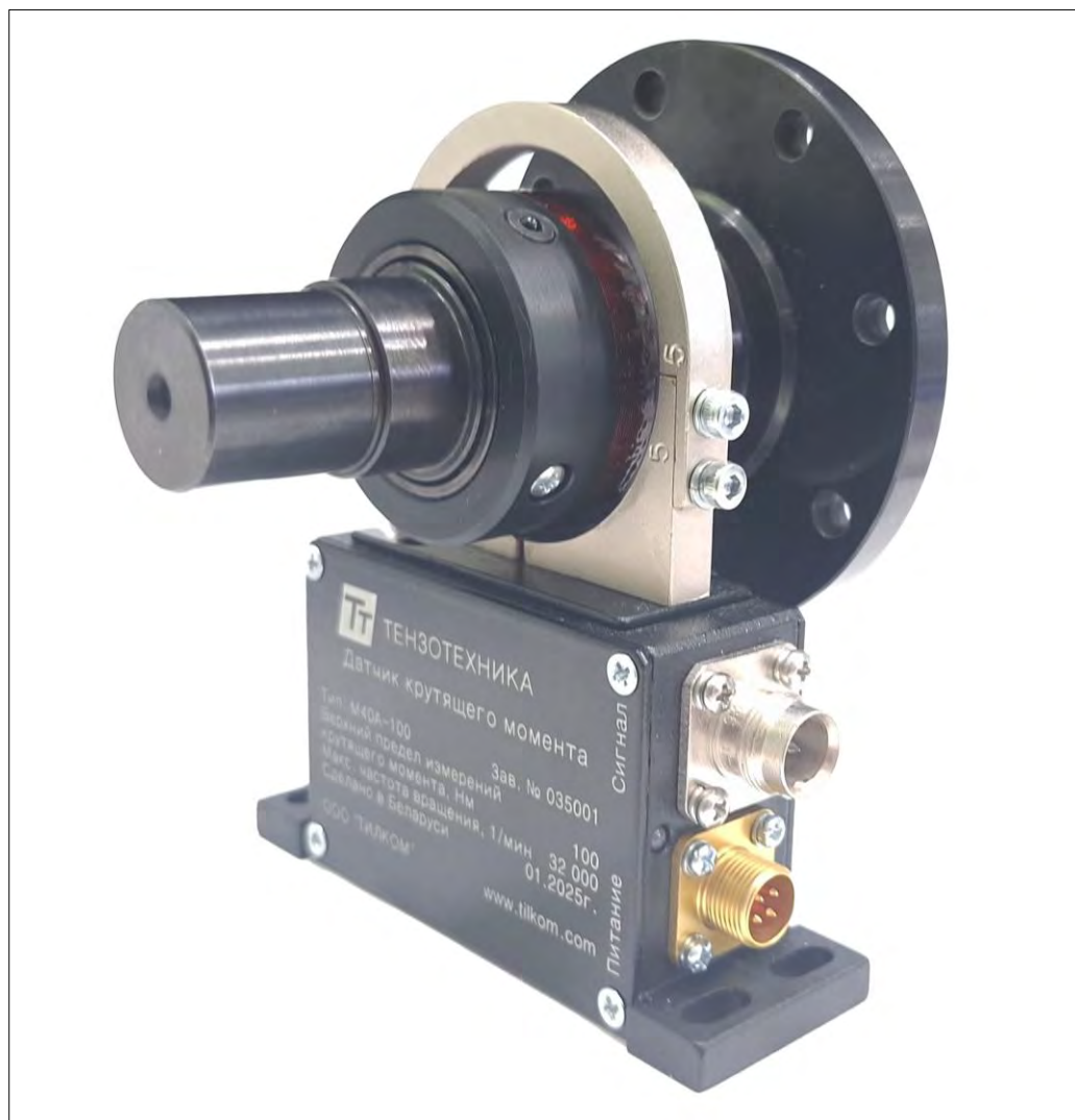
Рис. 1 – Внешний вид датчика М40А
