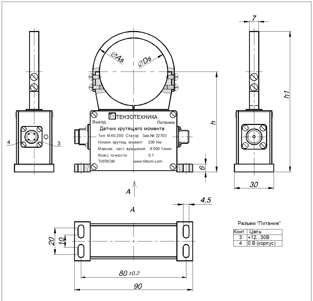
Рис. 6– Статор М40А-5... М40А-300. Габаритные и установочные размеры, мм
