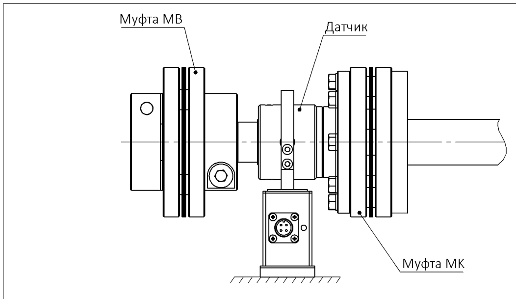
Рис. 9 – Установка датчика М40А с применением дисковых компенсационных муфт МВ и МК
