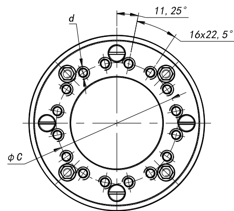
Располож. крепежн. отв. D
