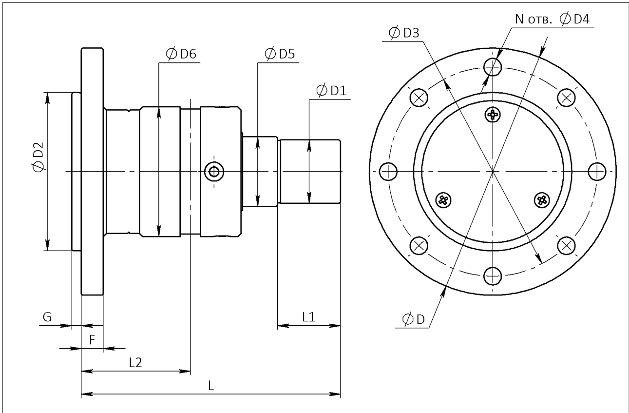
Рис. 5 – Ротор М40А. Габаритные и установочные размеры, мм
