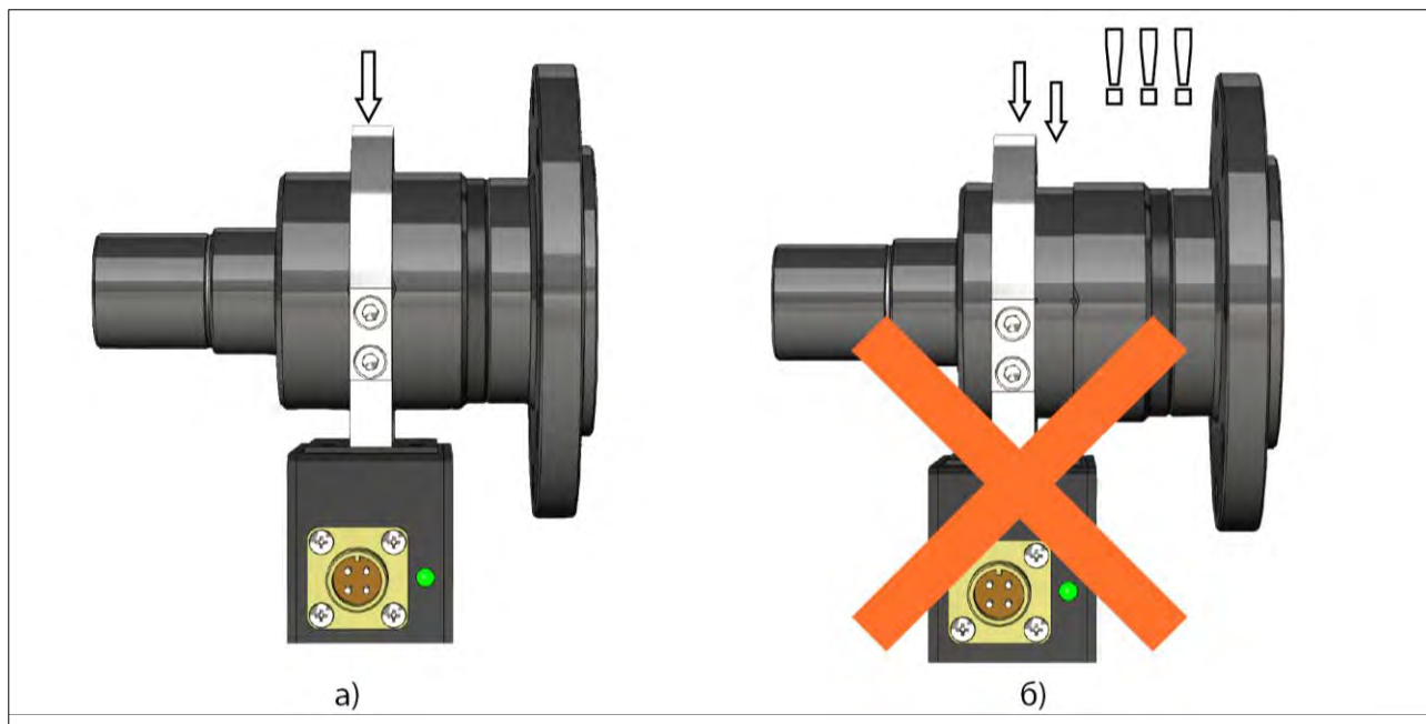
Рис. 11 – Расположение кольца статора относительно катушки ротора: а – ПРАВИЛЬНОЕ, б – НЕПРАВИЛЬНОЕ
